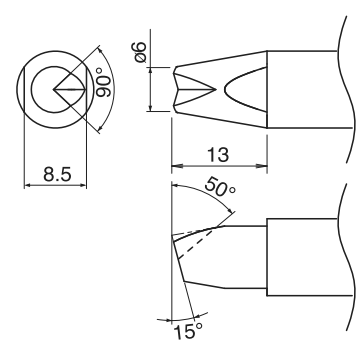
TX2-XBCR6 6XBC型 帶 V 型槽
