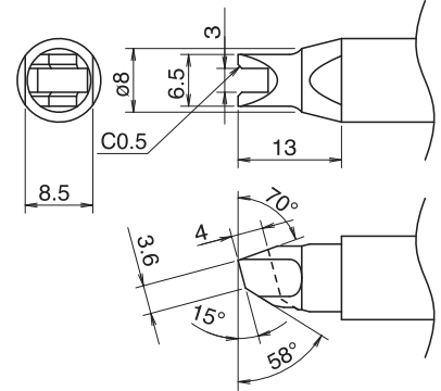
TX2-XRK3065 XK型 帶凹面 內溝 3.0 / 外圍 6.5 / 深度 4.0 mm
