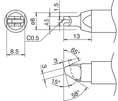
TX2-XRK1545 XK型 帶凹面 內溝 1.5 / 外圍 4.5 / 深度 3.0 mm
