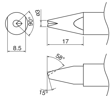
TX2-XBCR3 3XBC型 帶 V 型槽
