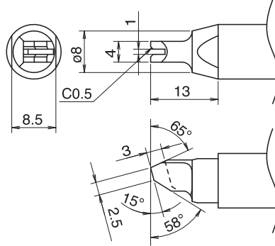
TX2-XRK1040 XK型 帶凹面 內溝 1.0 / 外圍 4.0 / 深度 3.0 mm
