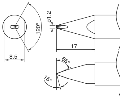
TX2-XDRF12* 1.2XD型 帶 V 型槽
