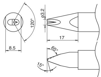
TX2-XDRF32* 3.2XD型 帶 V 型槽
