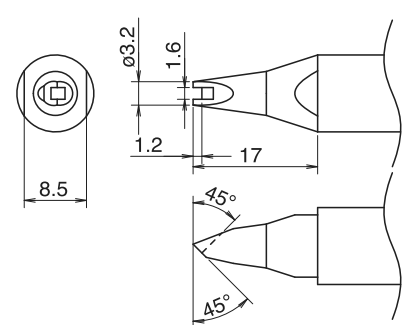
TX2-XDR1632 XD型 帶 V 型槽 內溝 1.6 / 外圍 3.2 mm
