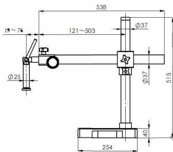
SZ-STL2 支架
