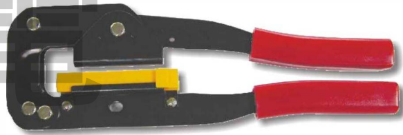
●最寬：55mm ●高度：6~27.5mm F 專利
